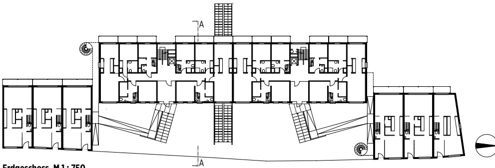
Erdgeschoss, M 1 : 750
