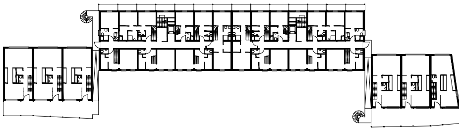
3. Obergeschoss, M 1 : 750
