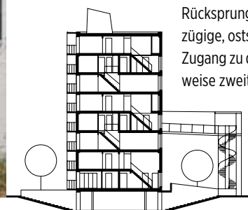
Schnitt A-A, M 1 : 750
