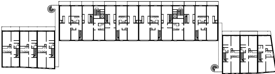
1. Obergeschoss, M 1 : 750
